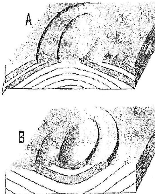
Figure 2.7 : Cuesta
